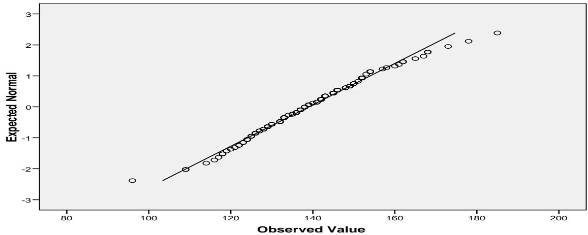
Normal Q-Q Plot of KonsepDiri
